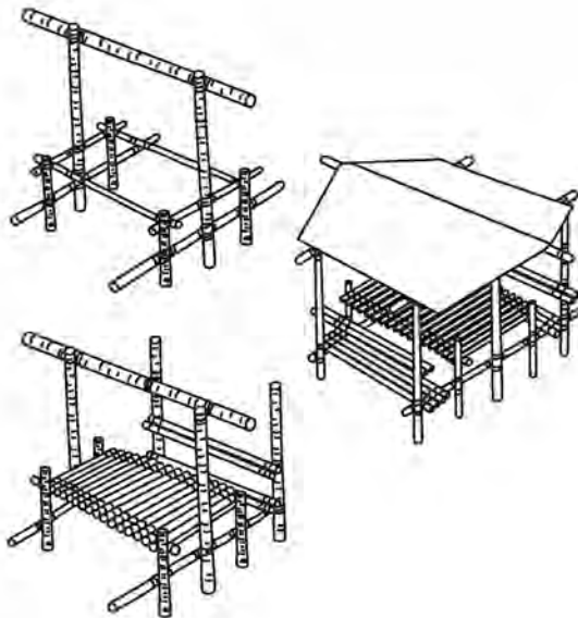
Rajah 13.19: Gajet tempat berteduh
