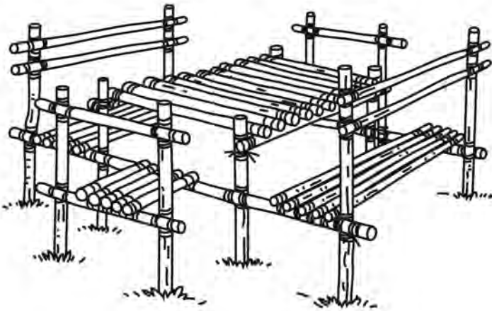
Rajah 13.7: Gajet meja makan
