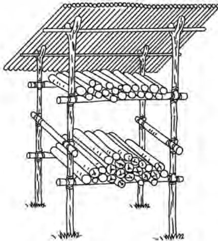
Rajah 13.9: Gajet menyimpan kayu api
