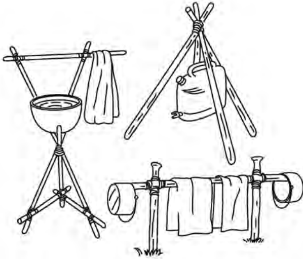
Rajah 13.8: Gajet penyangkut cawan / gelas
